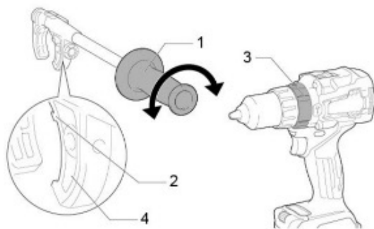
1. Рукоятка 2. Паз
